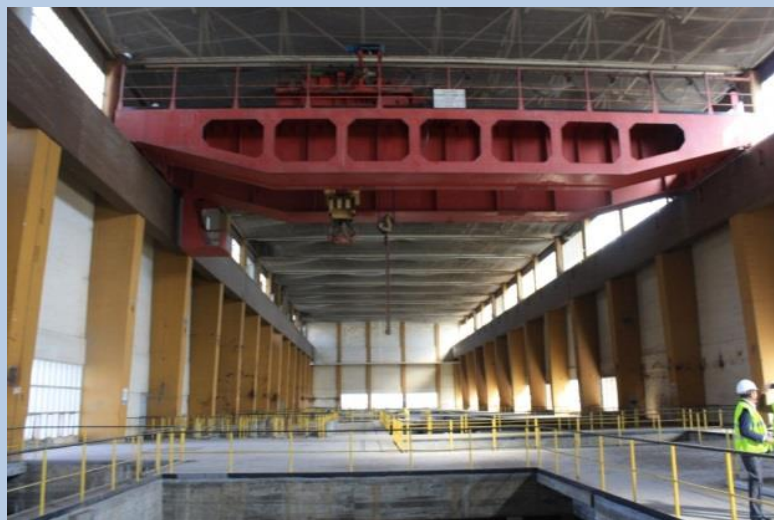
Edificio de Turbinas, última planta de 5,600 m 2 en su estado actual
